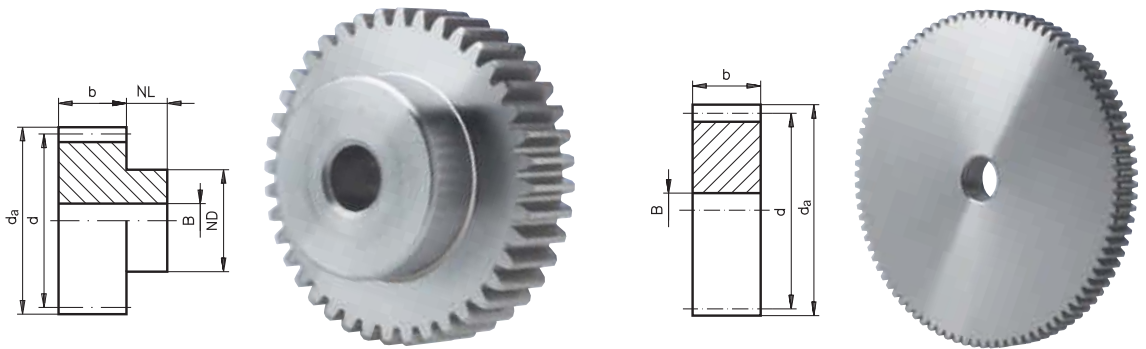
Modul 2,0 – Zahnbreite: 20 mm mit Nabe
