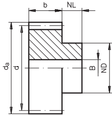
Modul 2,5 – Zahnbreite: 25 mm mit Nabe
